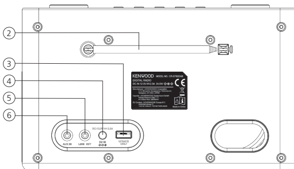
Lato posteriore
